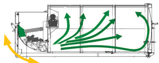
Schwingkolbenpresse für Naßabfälle
