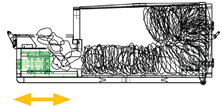
Stempelpresse für Trockenabfälle
